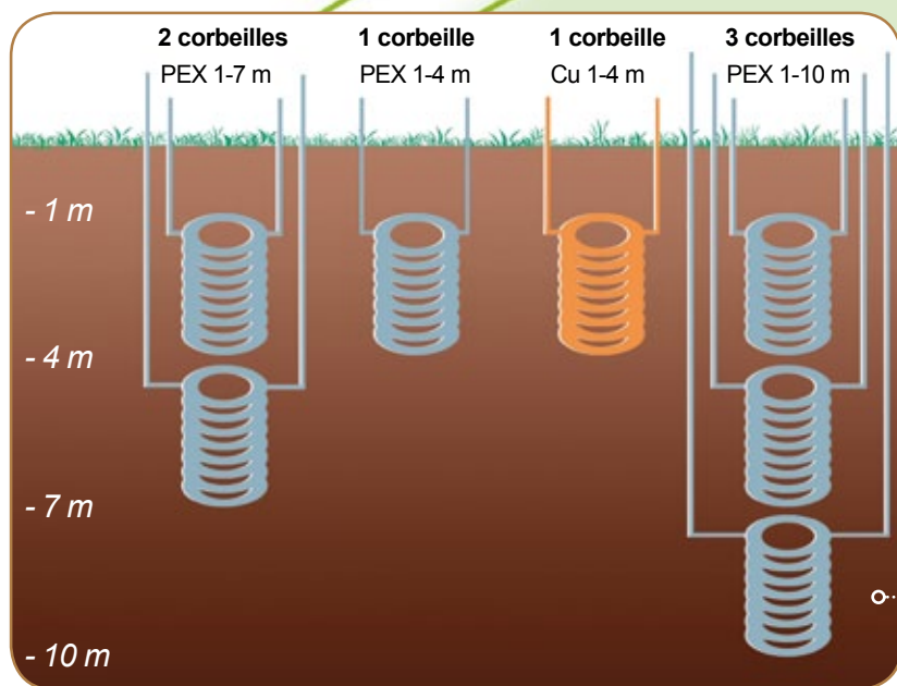
Vue en coupe de l'implantation de corbeilles géothermiques
